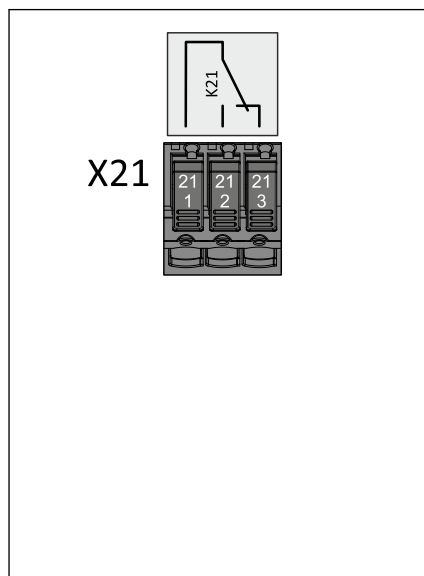
Bezpotencjałowy styk przekaźnika K21
