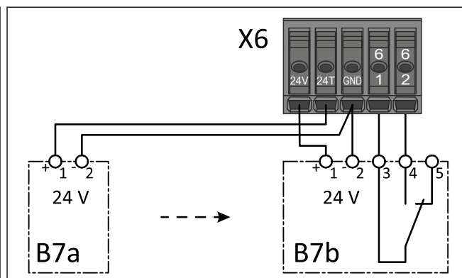
Fotokomórka jednokierunkowa, styk przełącznika wewnętrzny
