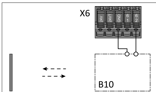
Fotokomórka refleksyjna dwużyłowa wewnętrzny
