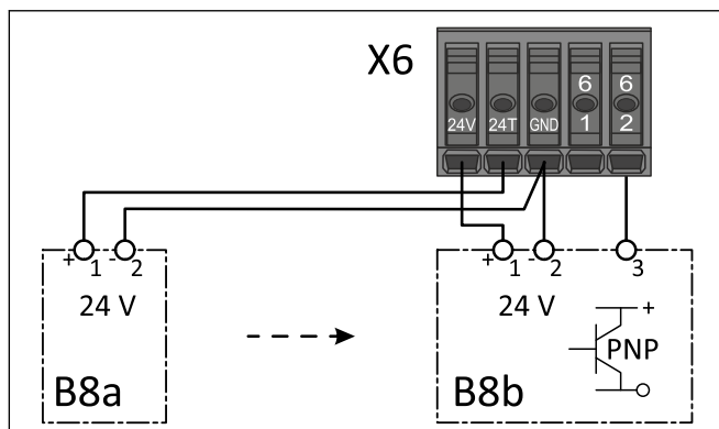
Fotokomórka jednokierunkowa, wyjście PNP wewnętrzny
