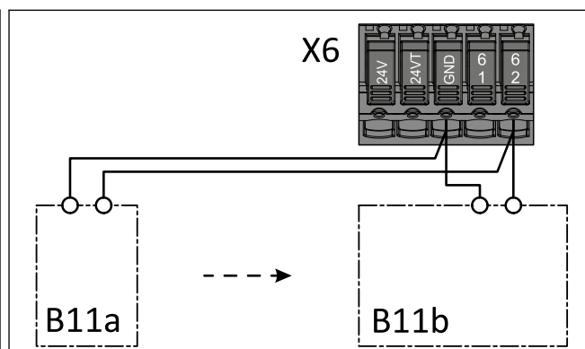
Fotokomórka jednokierunkowa dwużyłowa wewnętrzny
