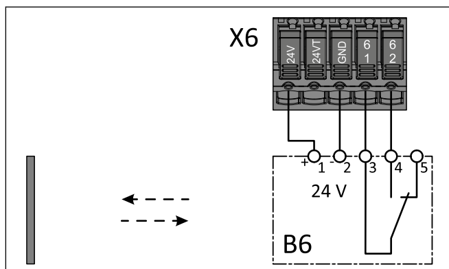
Fotokomórka refleksyjna, styk przełącznika wewnętrzny
