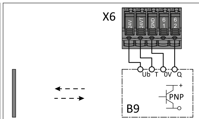
Fotokomórka refleksyjna testowana, wyjście PNP wewnętrzny
